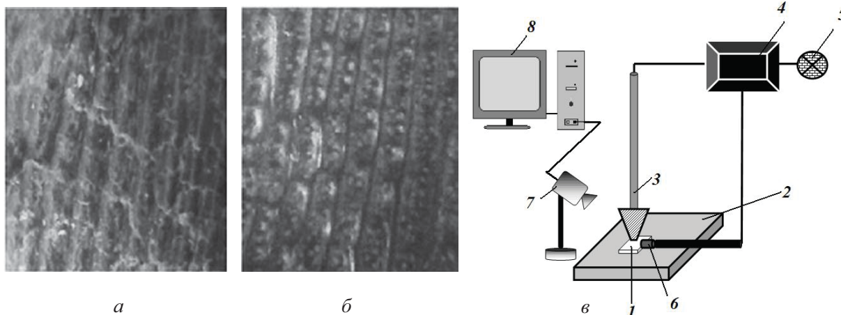
Рис. 1. Внешний вид обезвоженного (а) и насыщенного водой (б) образцов рогового слоя (увеличение в 5 раз), а также лабораторный стенд (в), содержащий: 1 – образец; 2 – неподвижную основу; 3 – электрод с медной насадкой; 4 – цифровой терморегулятор; 5 – источник питания; 6 – термодатчик; 7 – видеокамеру; 8 – компьютер
